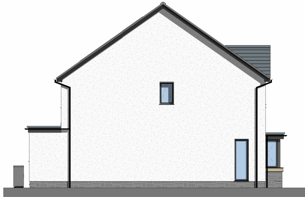
SIDE. 1 : 100
