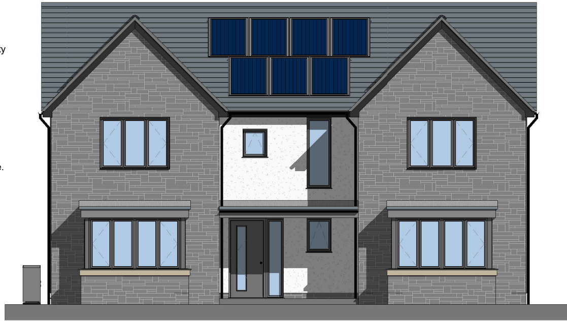
FRONT 1 : 100
