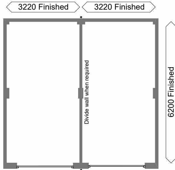
PLAN 1 : 100
