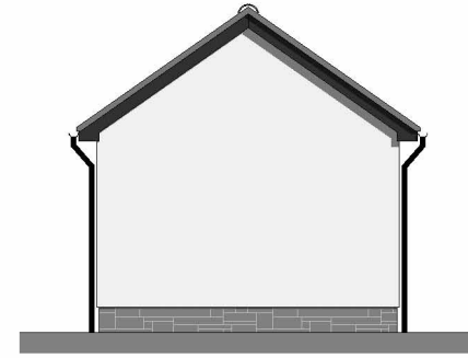
REAR 1 : 100
