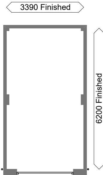
PLAN 1 : 100
