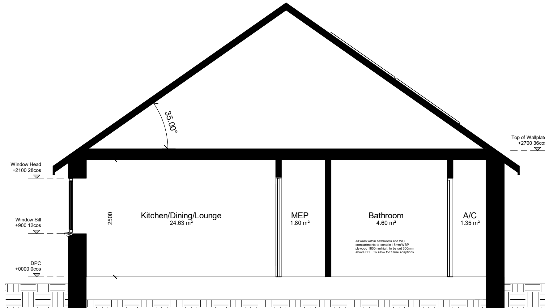
Section 1 : 50
